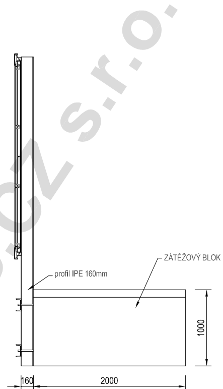
ŘEZ 1
