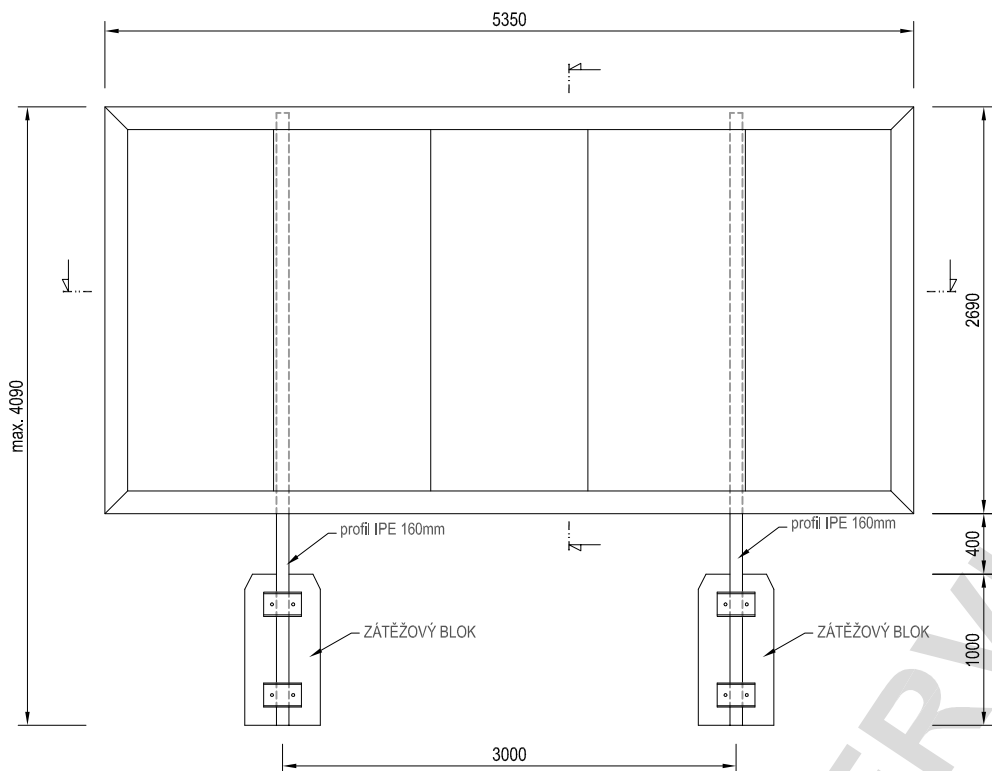
POHLED ČELNÍ
