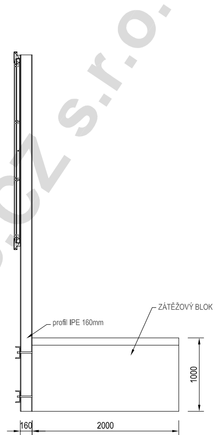
ŘEZ 1
