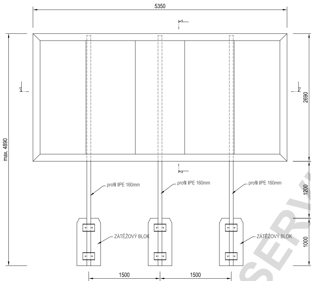
POHLED ČELNÍ
