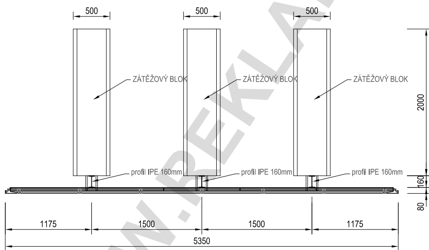
ŘEZ 2
